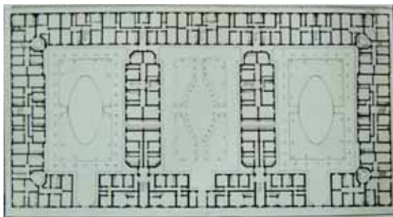
Pianta del 9° blocco di case popolari a Firenze: 14 fabbricati con 272 appartamenti, realizzato nella zona di Coverciano fra le vie Manni, d'Orso e Gelli fra 1929 e 1931, disegno di Carlo Burci
